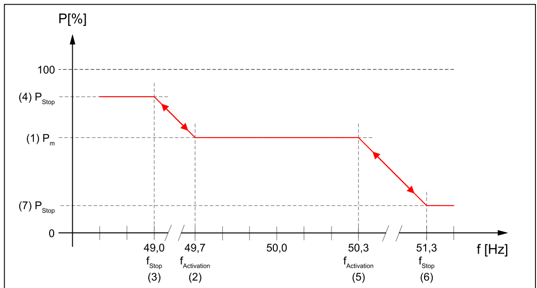
Curva general de potencia en caso de exceso y falta de frecuencia, sin histéresis y con frecuencia de parada.
